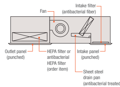
Diagram Struktur
