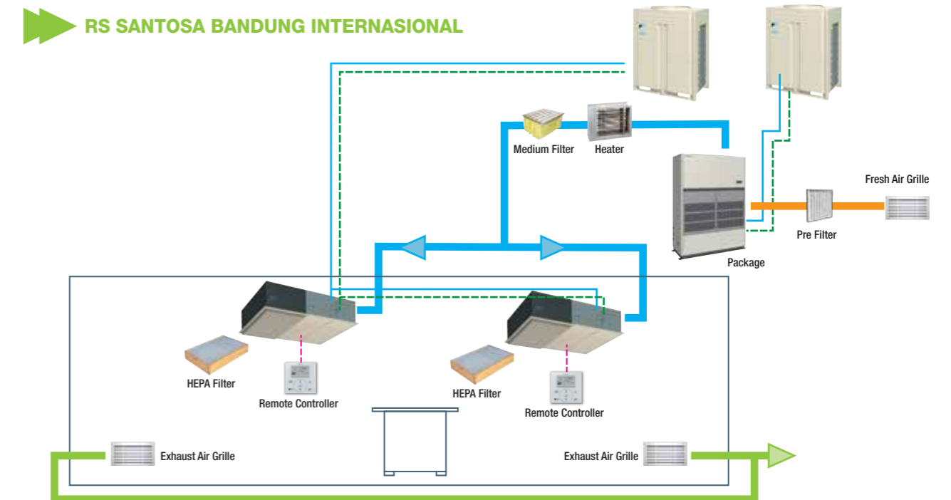
Gambar Skema
