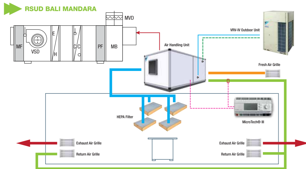
Gambar Skema
